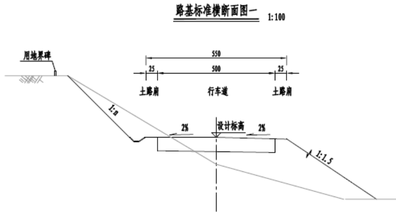
路基横断面图
