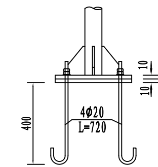
基础主筋大样图 1: 20
