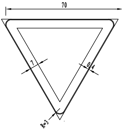
禁令标志1尺寸
