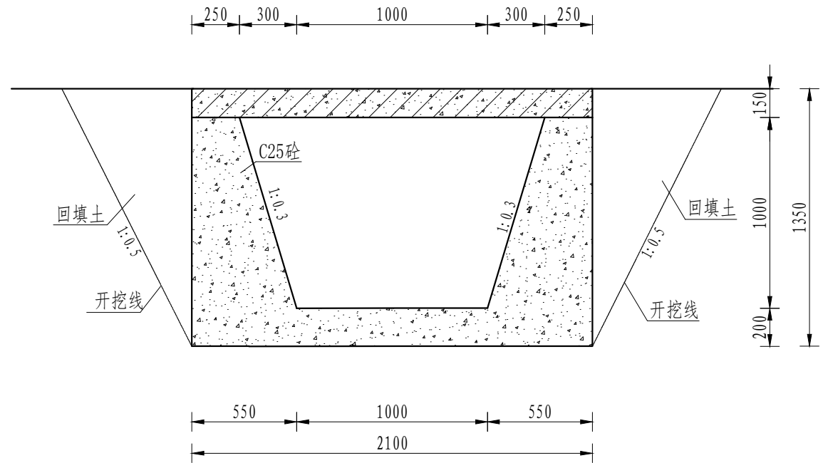
A-A剖面图 1:20
