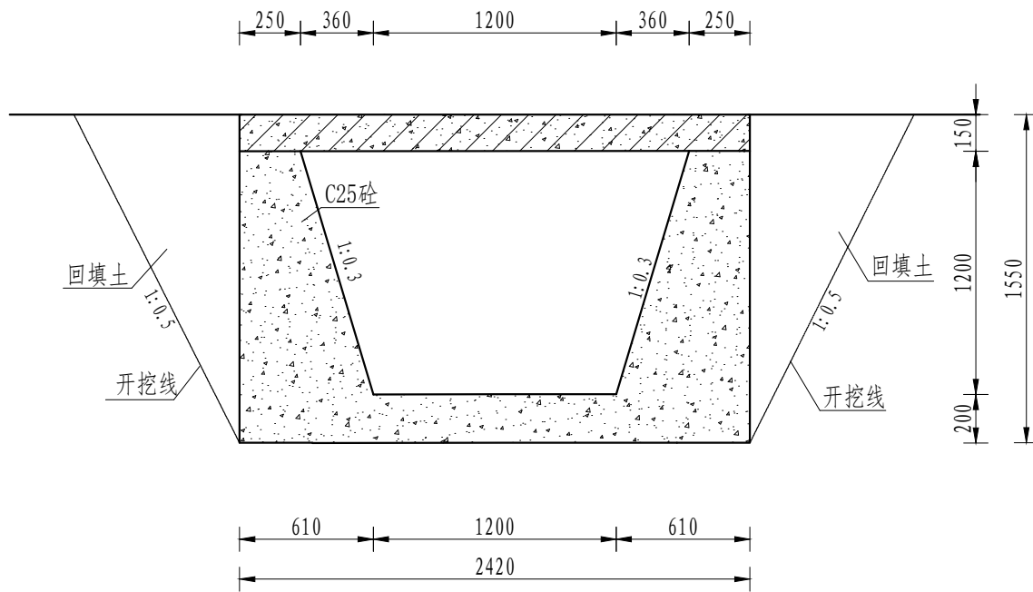
A-A剖面图 1:20
