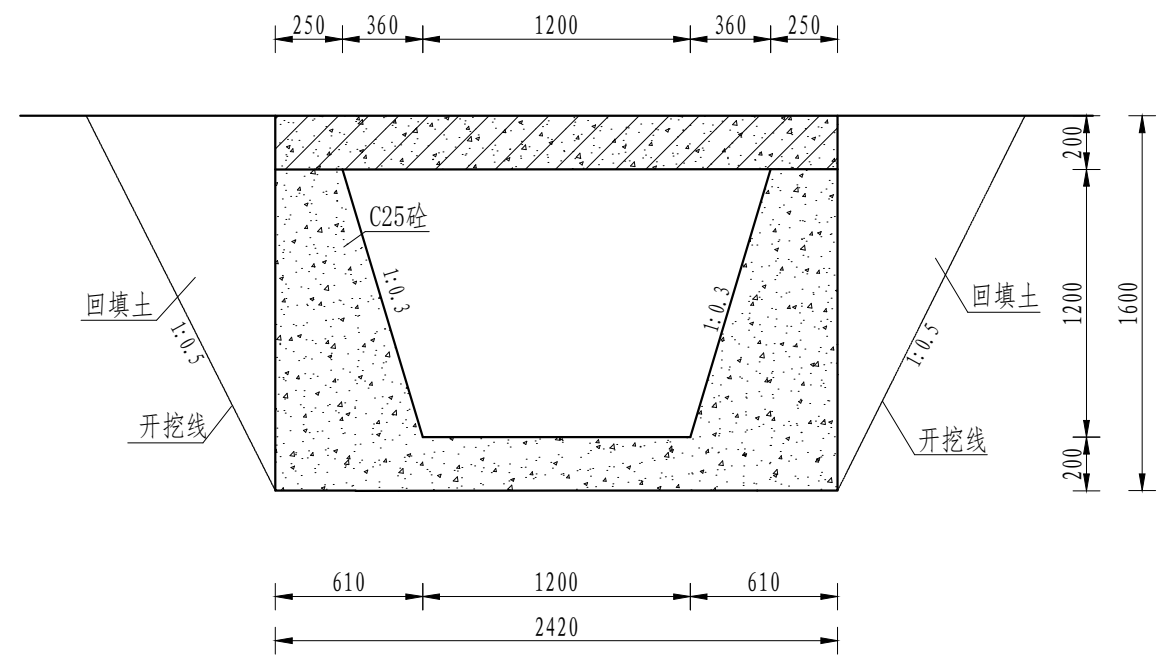
A-A剖面图 1:10
