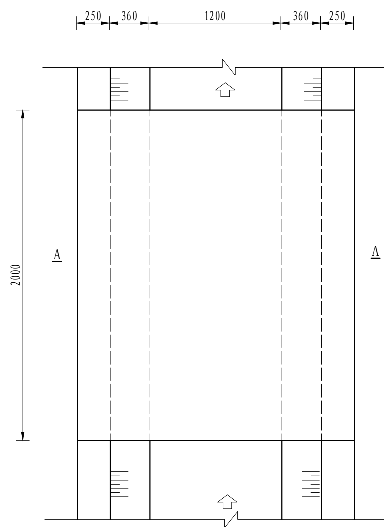
机耕桥板平面图 1:20
