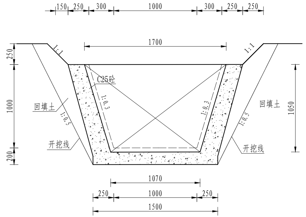
A-A剖面图 1:25
