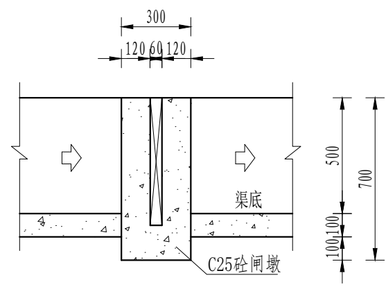
A-A剖面图 1:20
