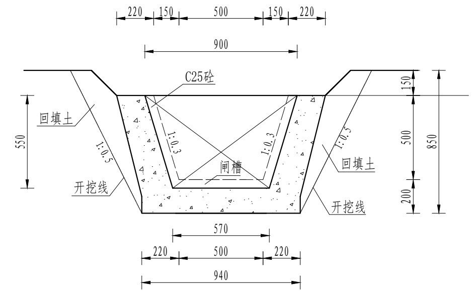
B-B剖面图 1:20
