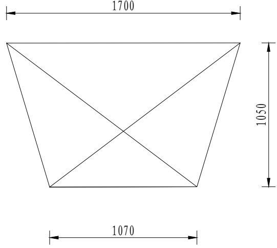
木闸门尺寸图 1:20
