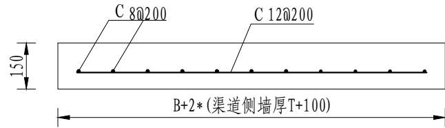
人行桥板配筋图 1:10
