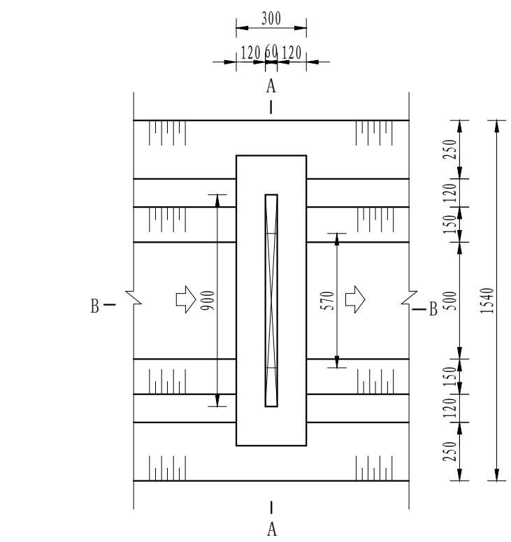
分水口平面图 1:20
