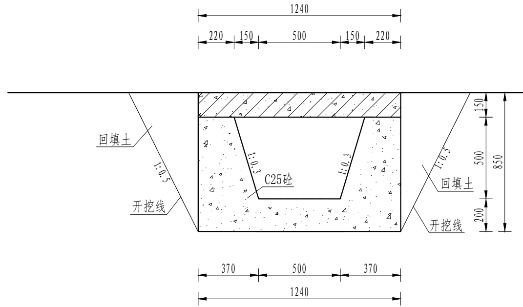
A-A剖面图 1:10
