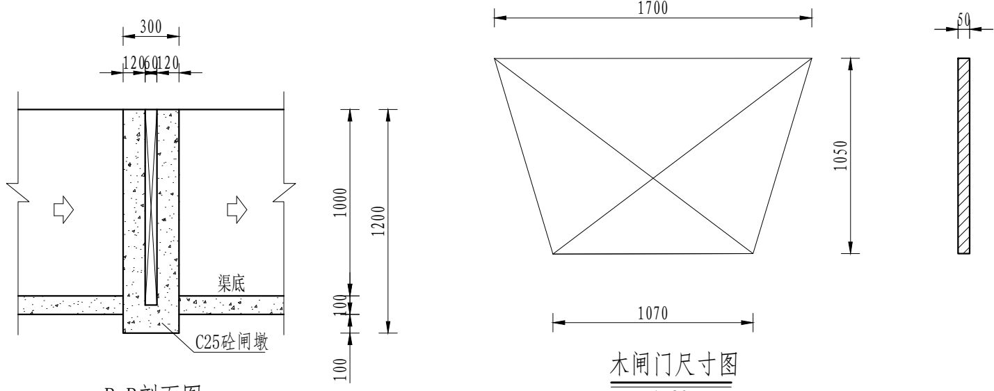
B-B剖面图 1:25
