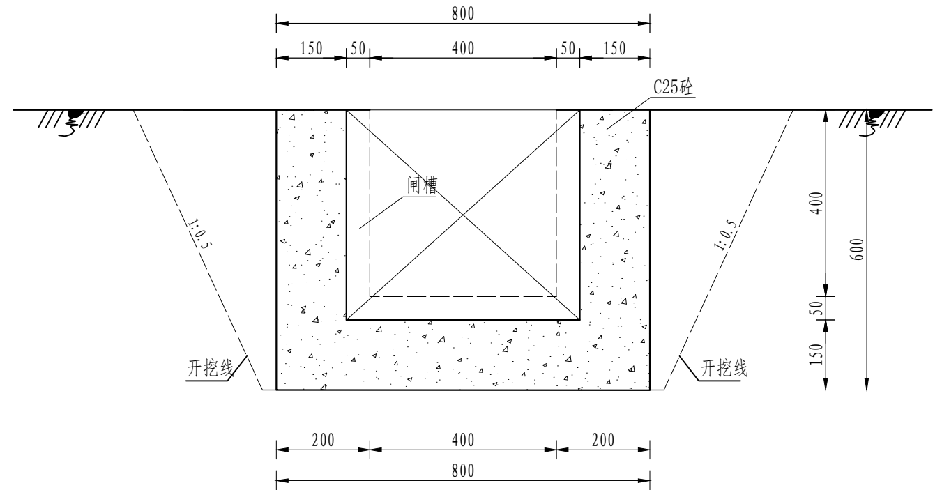
A-A剖面图 1:10
