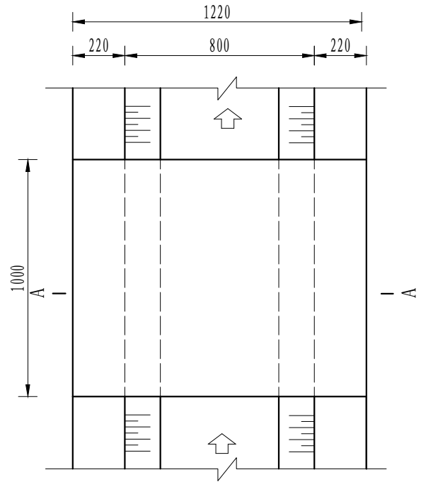
人行桥板平面图 1:20
