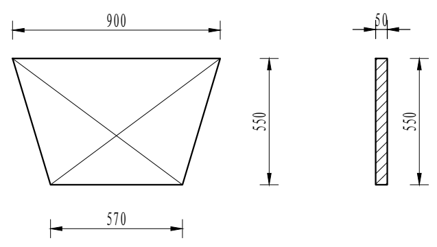
木闸门尺寸图 1:20
