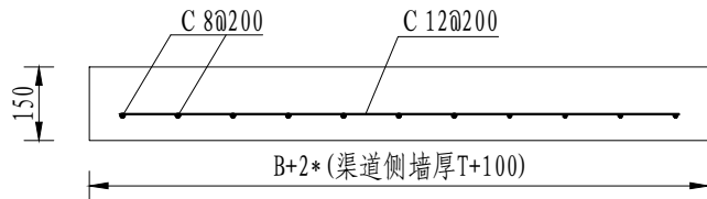
人行桥板配筋图 1:20
